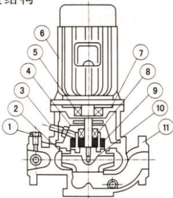
化工型结构
