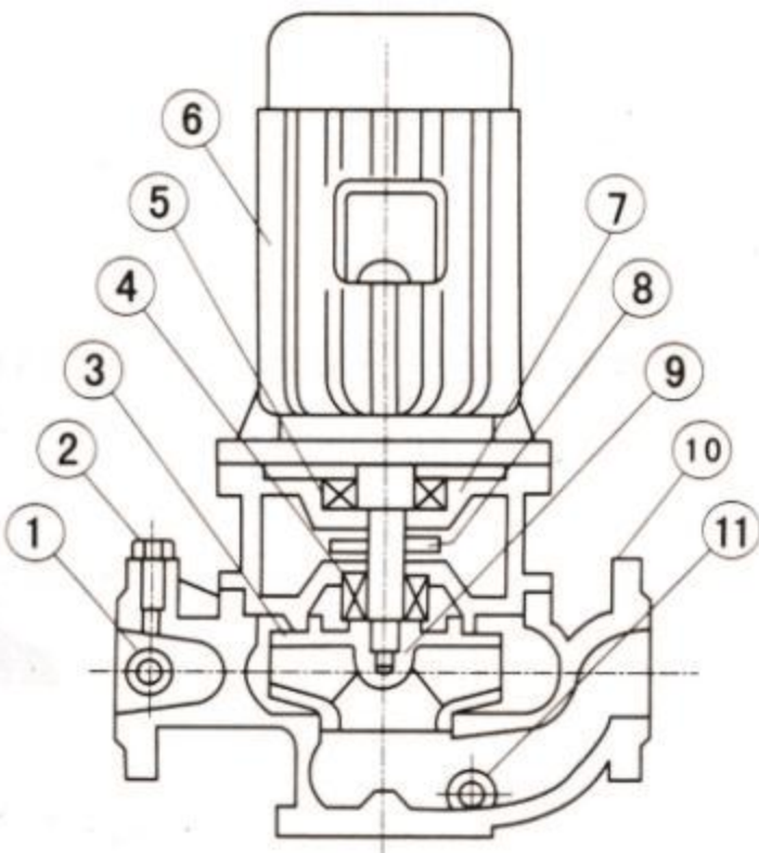
热水型结构
