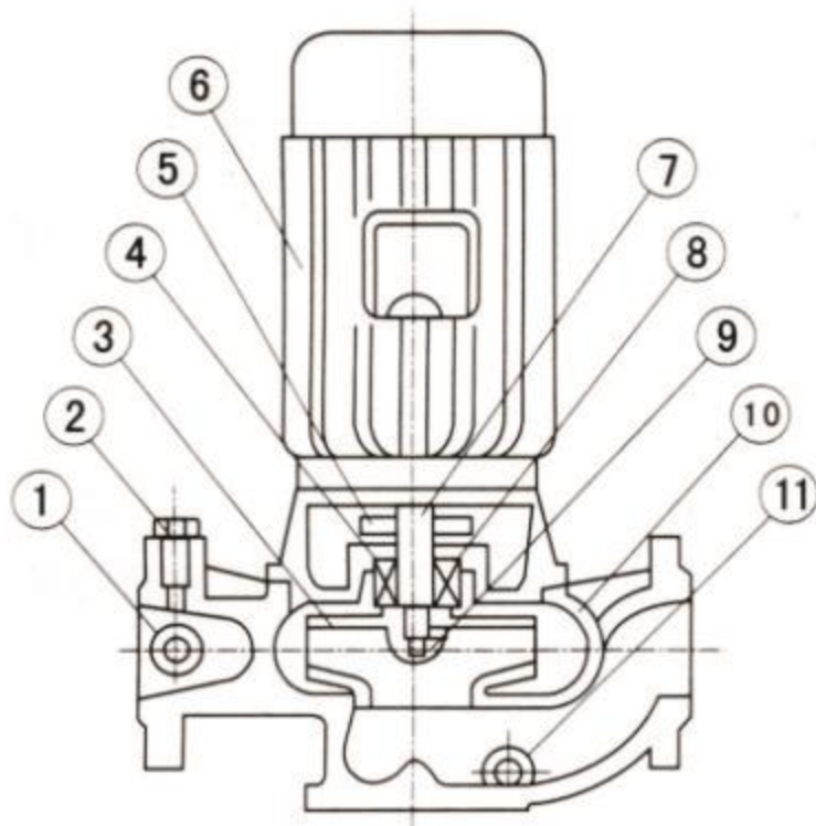
普通型结构
