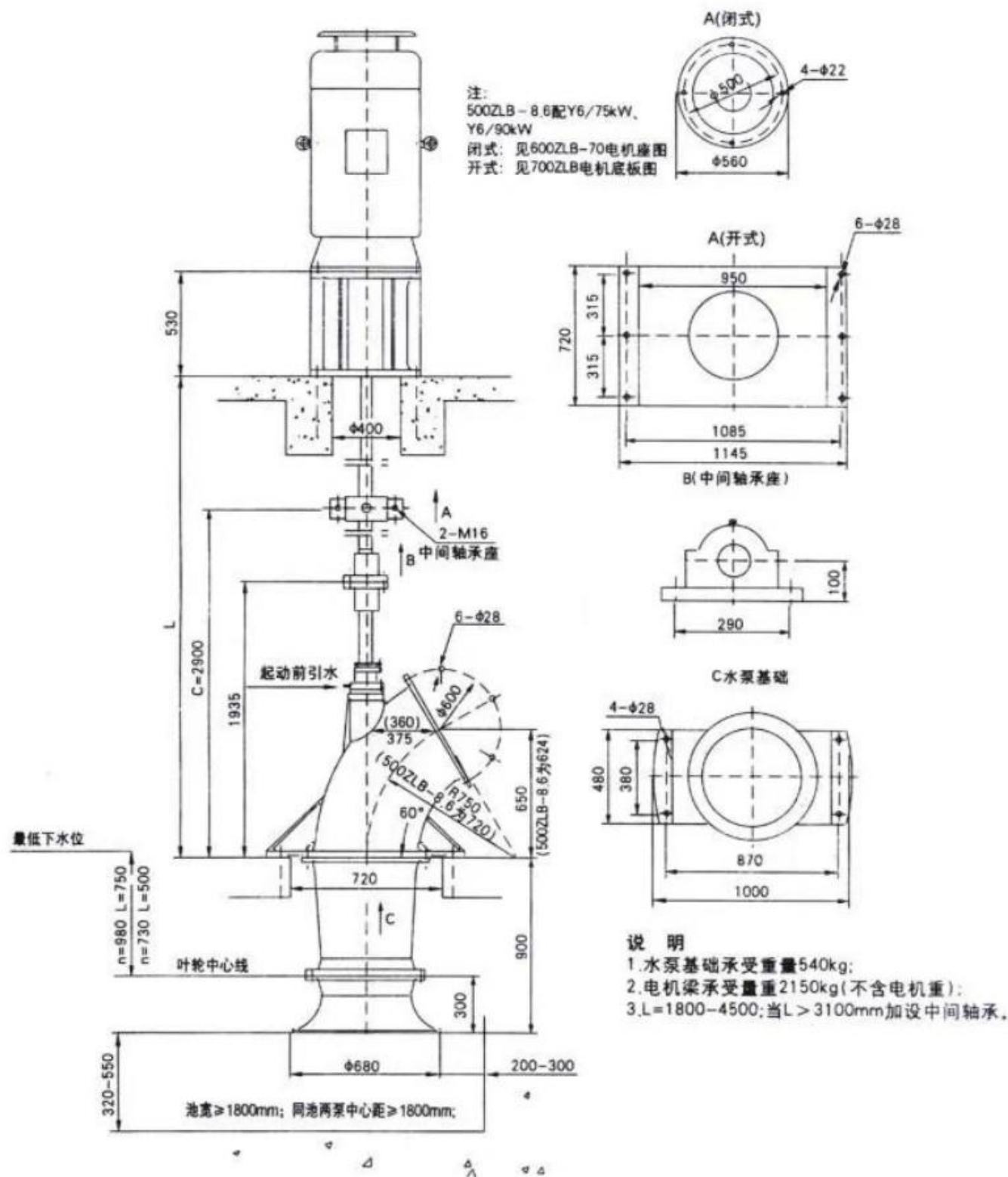
500ZLB 型轴流泵安装外形图
