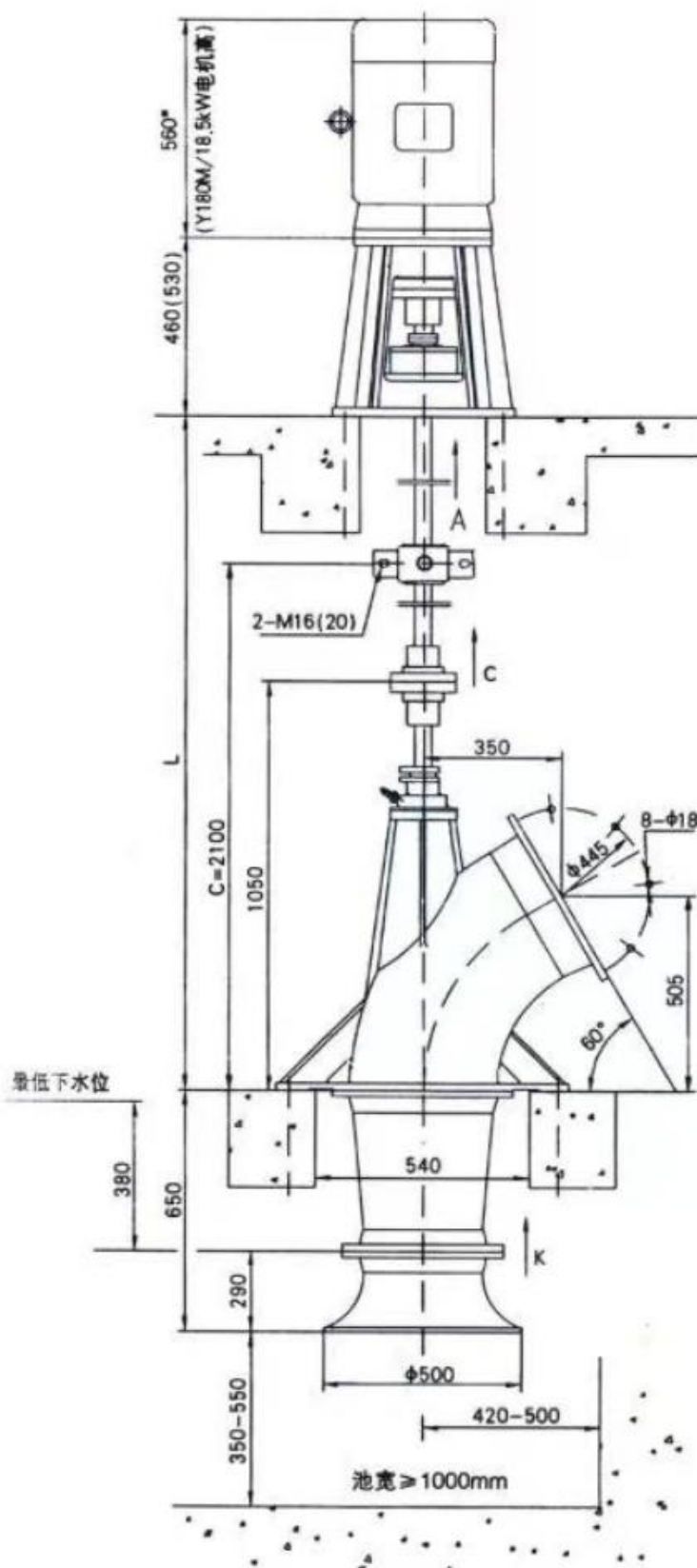
350ZLB型轴流泵安装外形图
